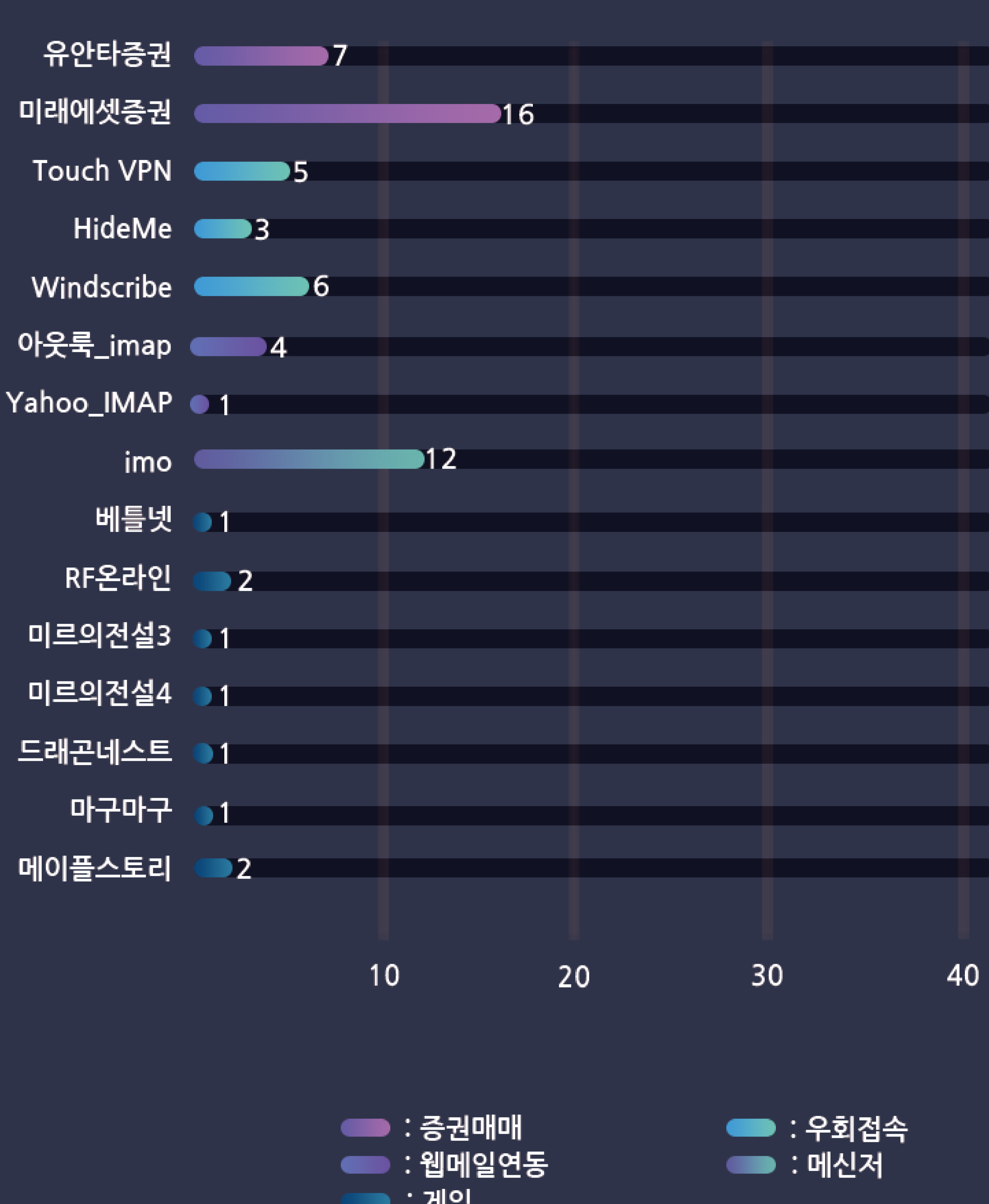
어플리케이션 추가된 패턴 수(IP/Port)
